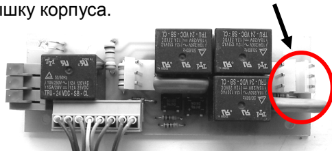
Рисунок 5. Релейный модуль Байпаса. Внешний вид
