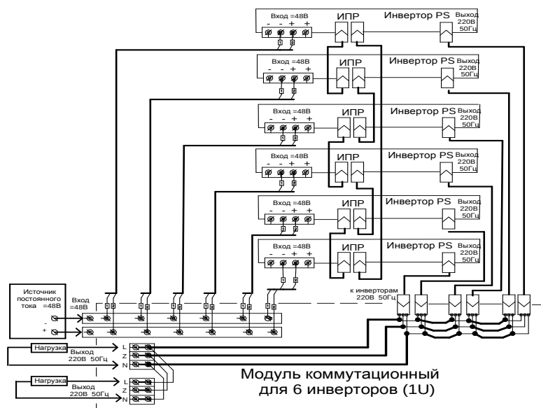
Типовая схема соединений с использованием 1U модуля коммутационного (1U) для 6 инверторов мощностью до 9 кВт.
