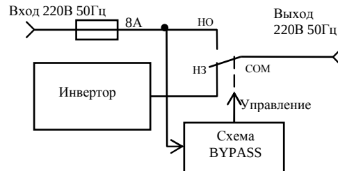
Рисунок 4. Основной источник – внешняя сеть (OFF LINE).
