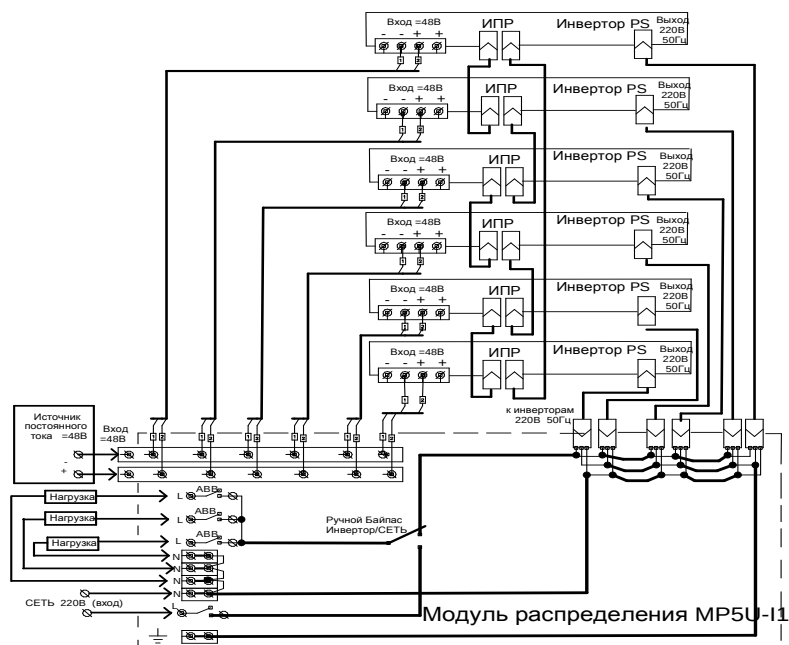
Типовая схема соединений с использованием 5U модуля распределения MP5U-11 с применением БАЙПАСА мощностью до 9 кВт.
